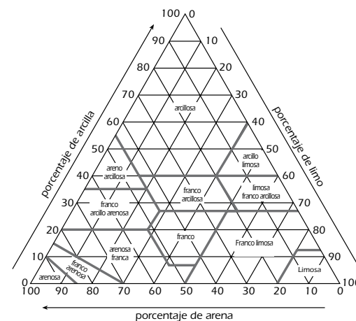
TRIÁNGULO DE TEXTURAS
