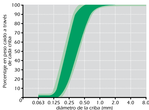
Curva granulométrica que define los límites recomendables y aceptables para sustratos de arena pura en campos de fútbol, rugby y hockey.
